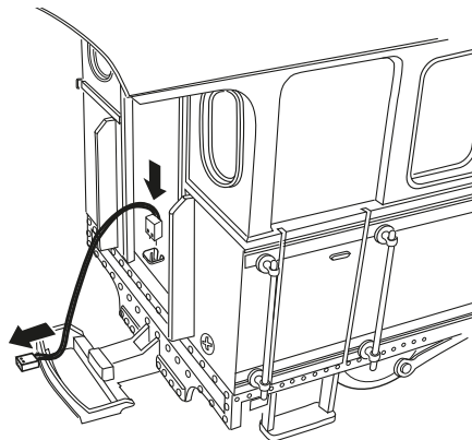
Bild 2, Verbindungskabel einstecken
